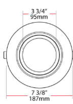
VISTA INFERIOR DE AMBAS LUMINARIAS
